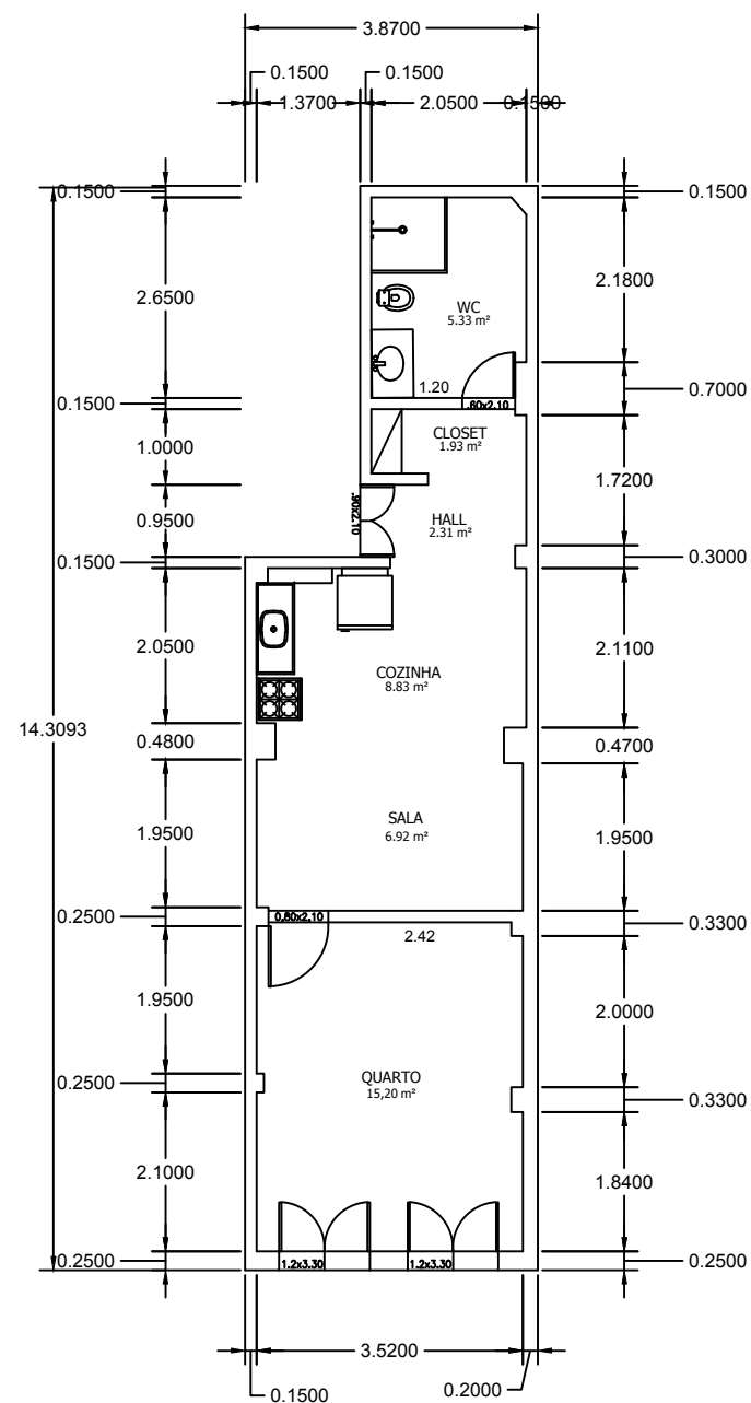
Planta Baixa - 1º Pavimento - Loft 03
