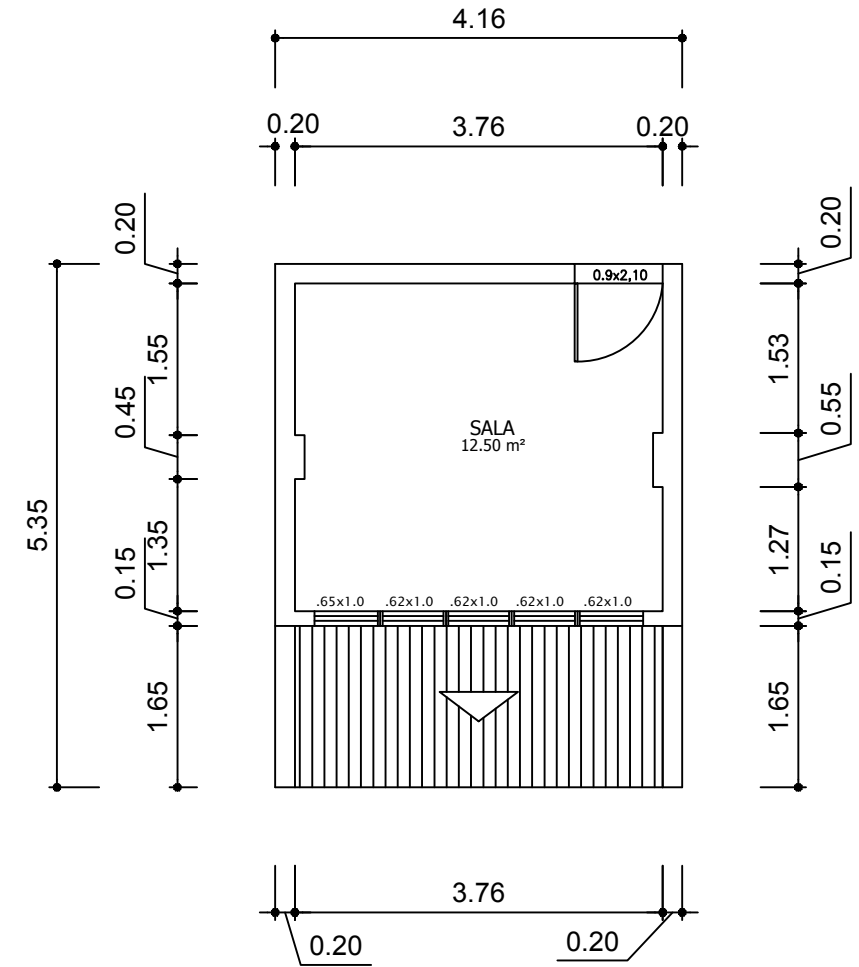
Planta Baixa - 1º Pavimento
